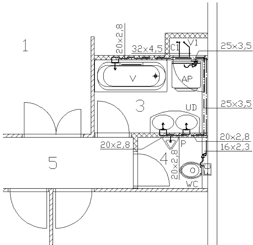
Obr. Ukázka řešení rozvodu vody
