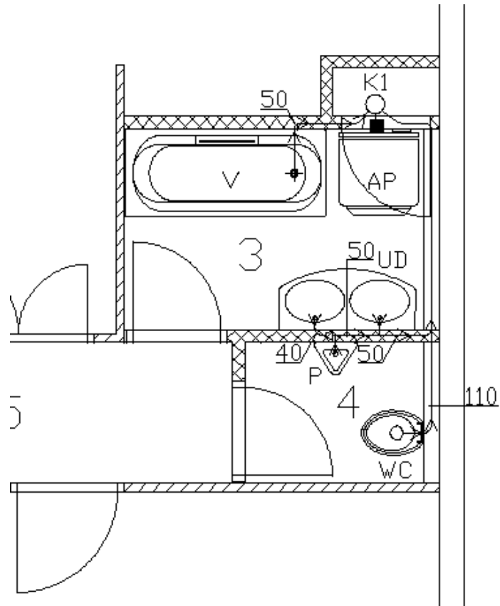
Obr. Ukázka řešení rozvodu kanalizace
