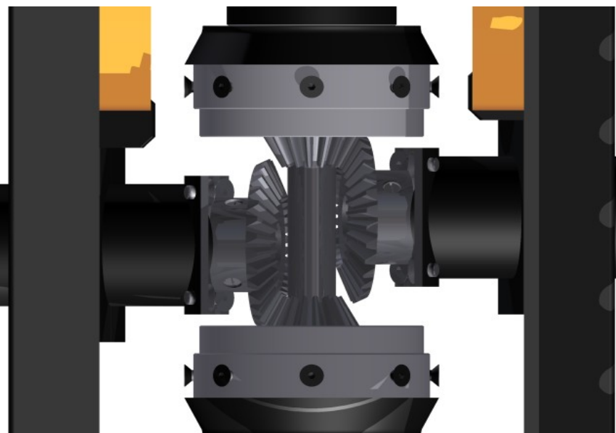
Obr. 2: Zjednodušení rozvodu na hnané zadní nápravě
